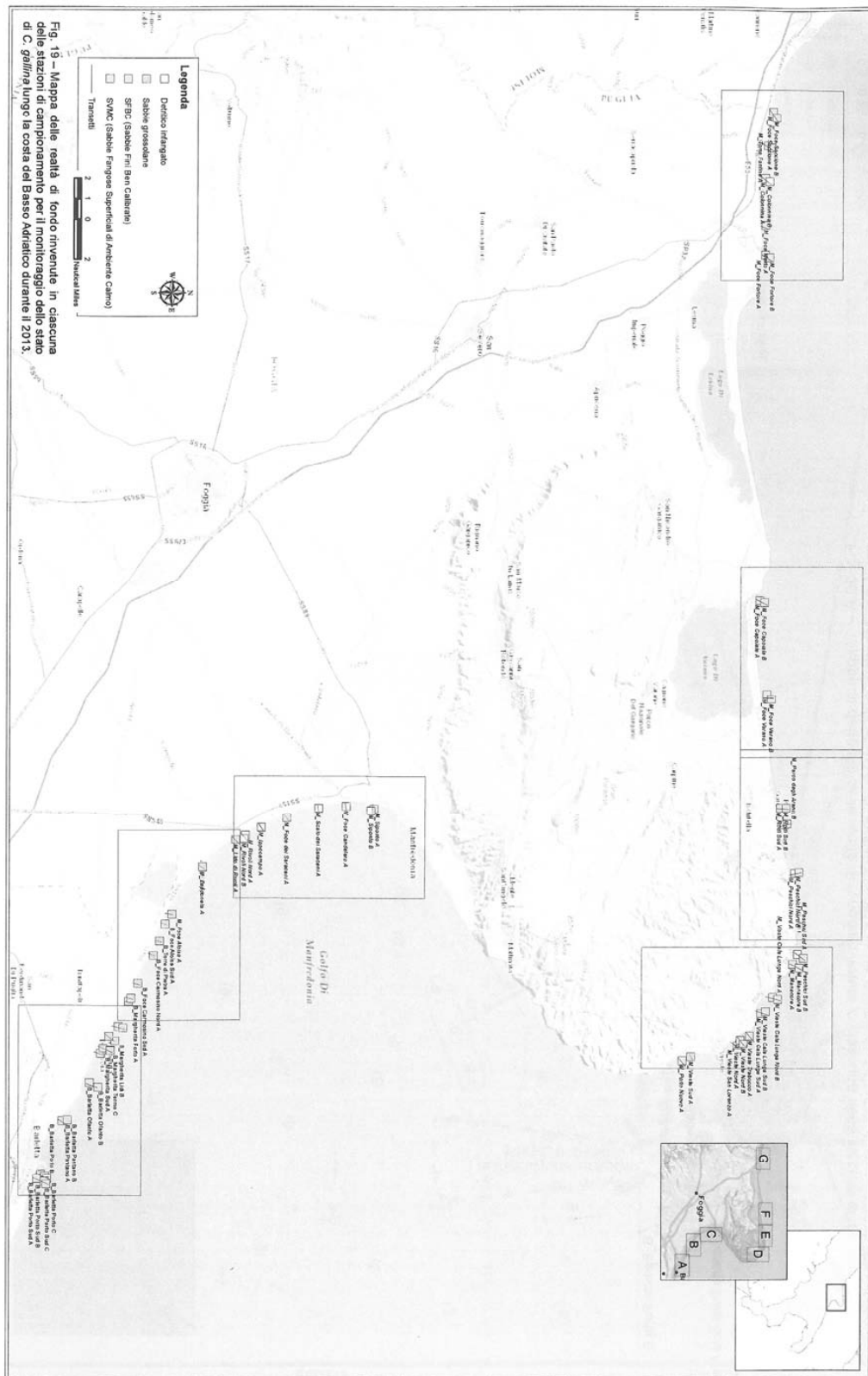
Fig. 39 – Mappa dei transetti nella Regione Puglia
