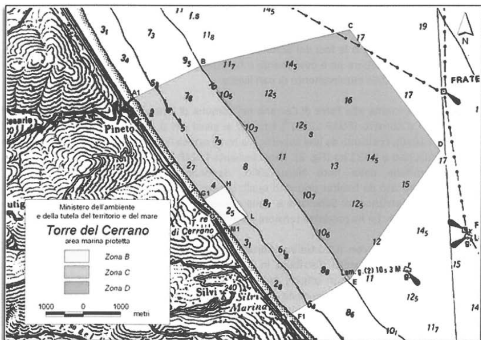
Figura 2. Planimetria dell'Area Marina Protetta "Torre di Cerrano".
