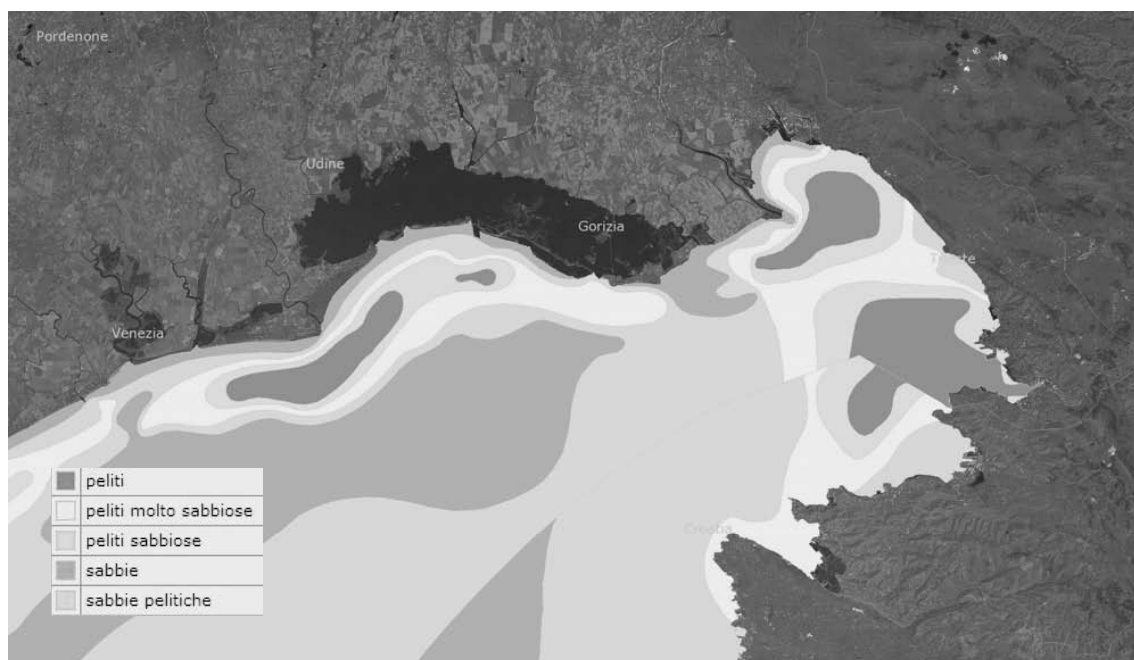
Fig. 2 - Carta sedimentologica dei fondali
