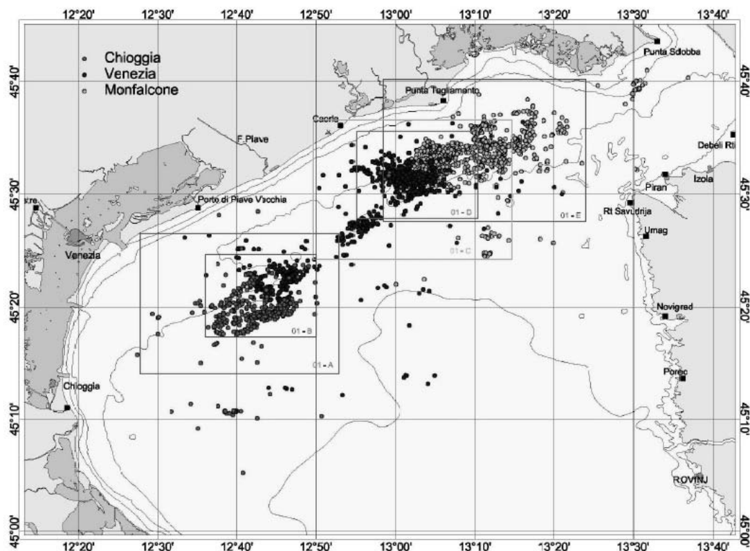
Fig. 3 - mappatura zone di pesca dei fasolari – Fonte O.P I Fasolari 2006
